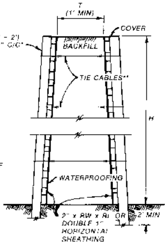
SECTION A-A
