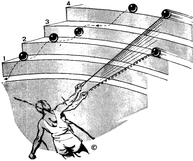
Fig. 26. THE QUANTUM LEAP
