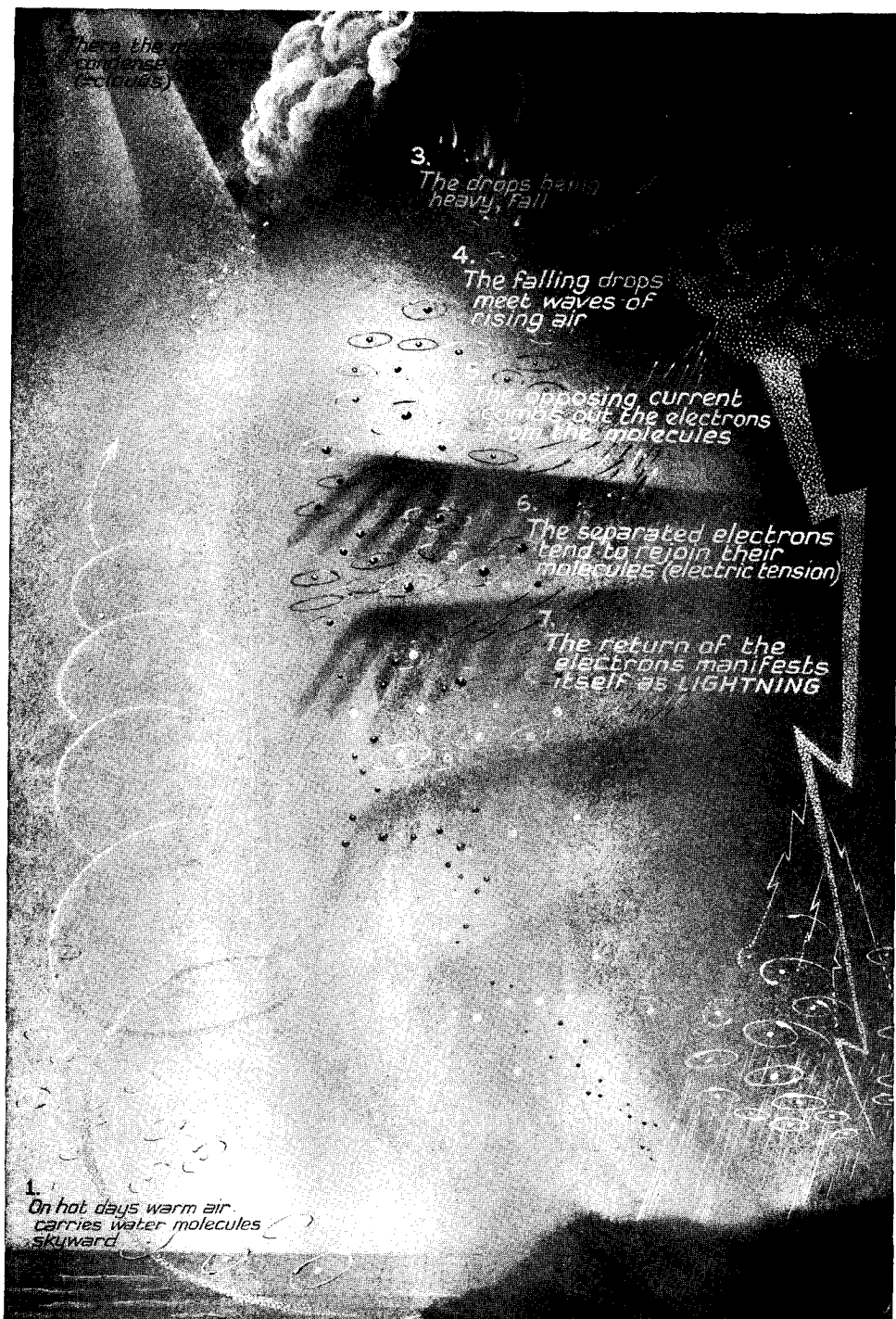
Fig. 123. THUNDERSTORM
