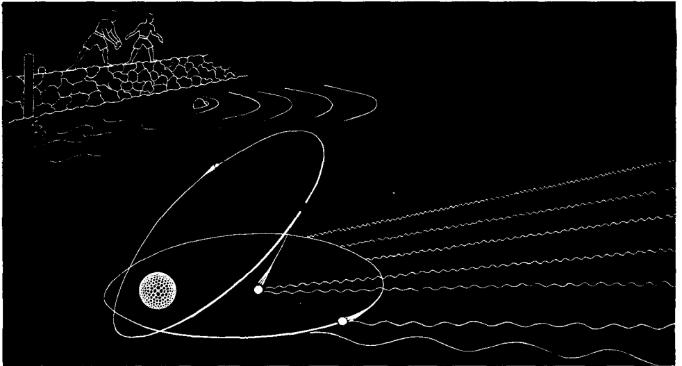
Fig. 22. WAVES
