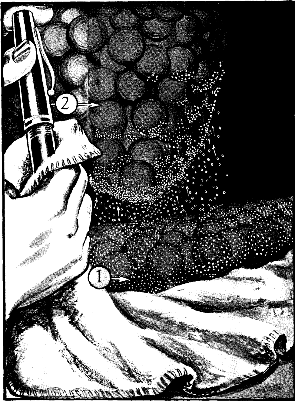
Fig. 14. ELECTRONS
