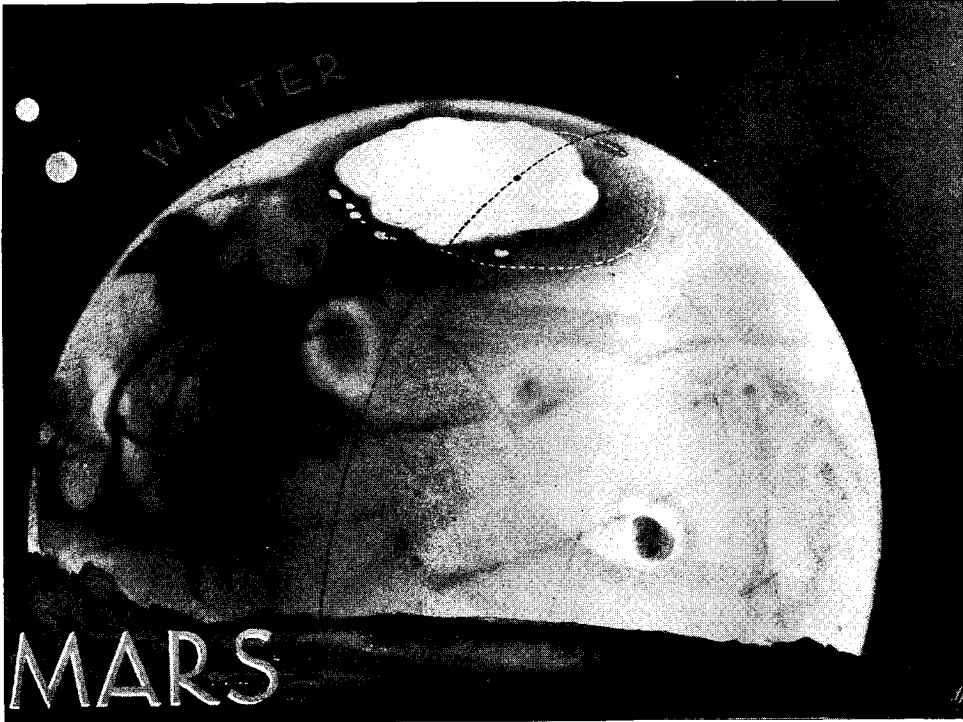
Fig. 82. MARS
