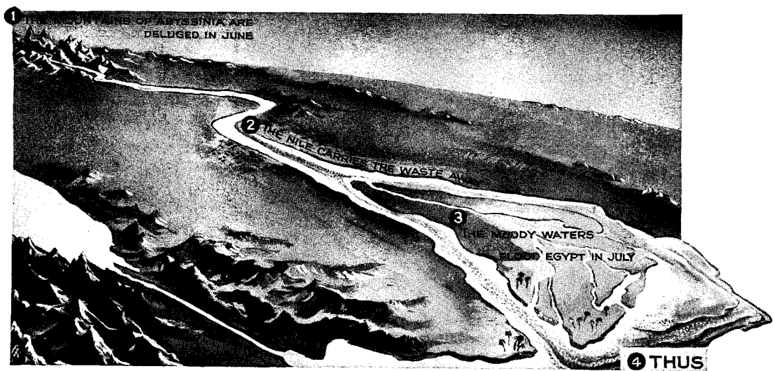
Fig. 138. DELTAS
