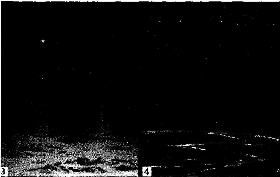
URANUS
