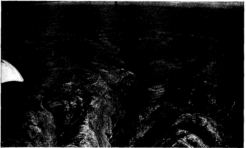
Fig. 146. EROSION
