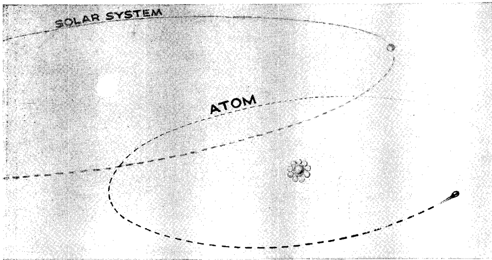
Fig. 13. THE ATOM
