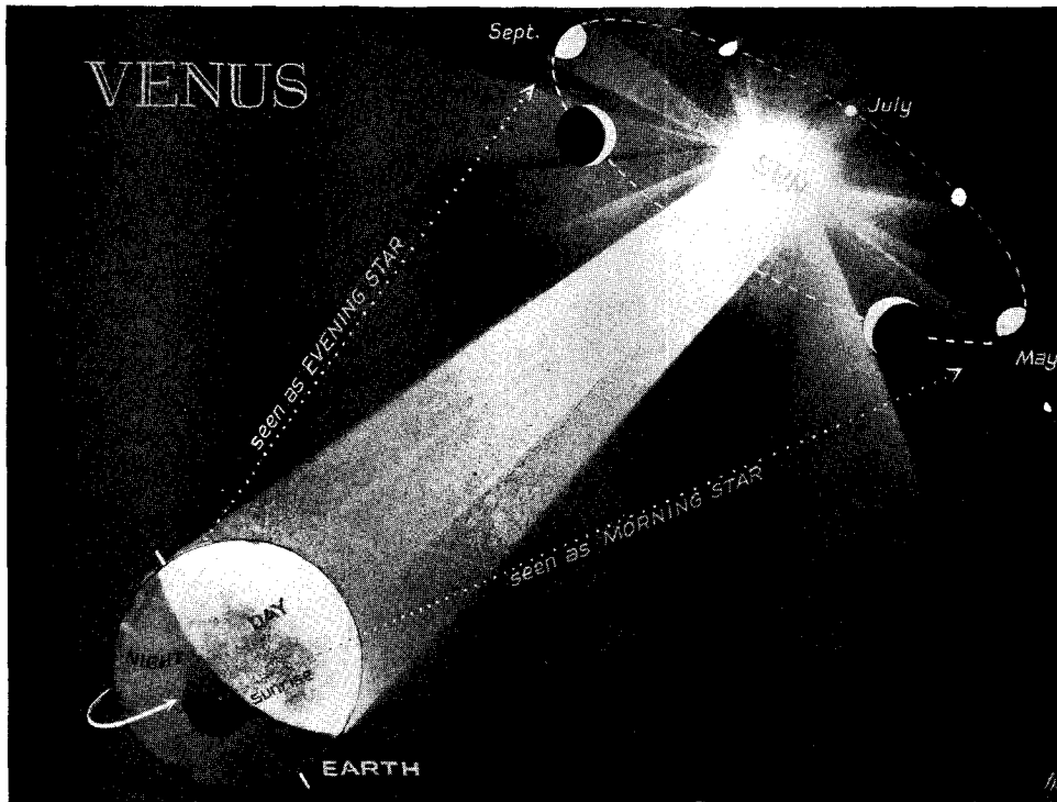
Fig. 81. VENUS
