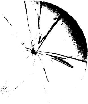
FIG. 3.—Codeine 1 : 50.
