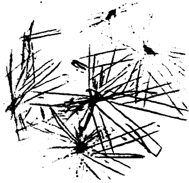
FIG. 6.—Hydrastinine 1 : 200.
