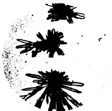
FIG. 1.—Narceine 1 : 50.
