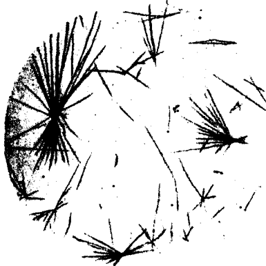
FIG. 4.—Berberine 1 : 500.
