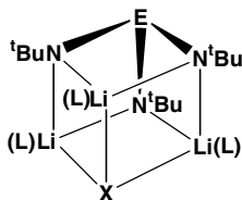
10.14 (E = S, Se)
