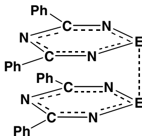
1.23 (E = S, Se)
