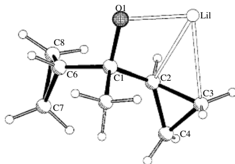
(17a)
