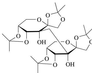
(271)
