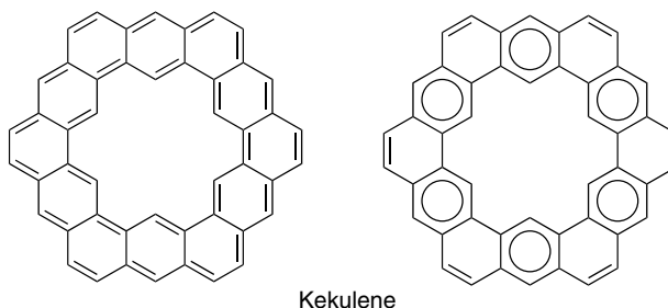
Kekulene
