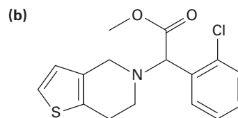
Clopidogrel (Plavix)
