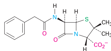
Benzylpenicillin
