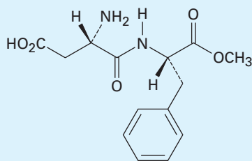
Aspartame
