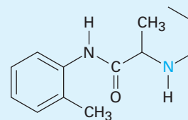
Prilocaïne (Citanest)
