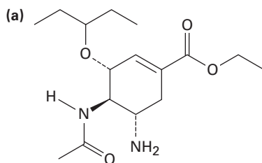
Oseltamivir (Tamiflu)
