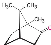
Camphor
