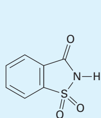
Saccharin
