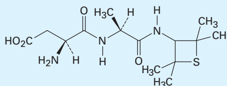
Alitame
