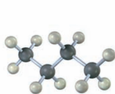
\text{CH}_3\text{CH}_2\text{CH}_2\text{CH}_3
