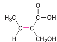
(Z)-2-Hydroxymethyl-2-butenic acid
