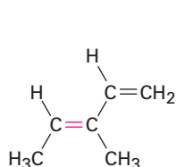
(E)-3-Methyl-1,3-pentadiene
