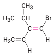
(E)-1-Bromo-2-isopropyl-1,3-butadiene
