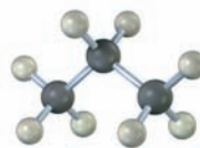
\text{CH}_3\text{CH}_2\text{CH}_3
