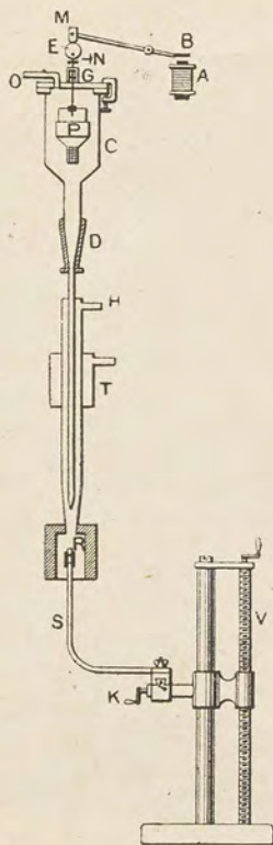
Abb. 1. Durchschnitt durch das von Verneuil zur Synthese des Rubins angewendete Gebläse.
