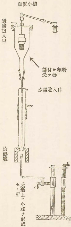
第二十二圖 ザエルヌイ式酸水素爐
