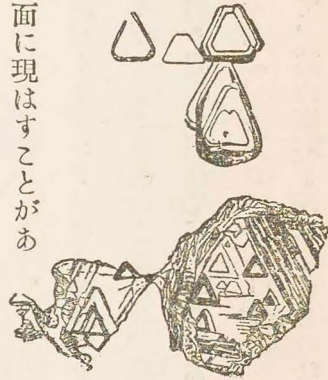
透明ダイヤモンドの内部に認められる三角形の線條 (約十八倍に擴大)
