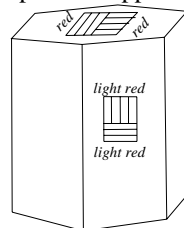
dichroismus of sapphire an optic uniaxial crystal
