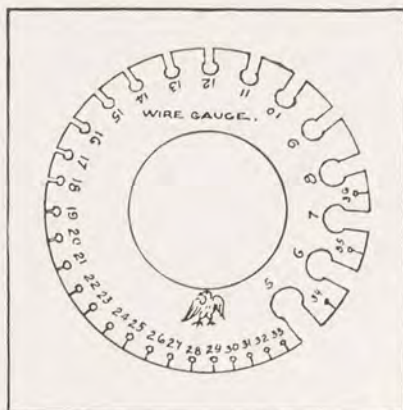
FIG. 8. THE WIRE GAGE
