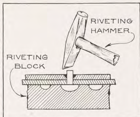
FIG. 112. RIVETING
