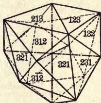
Fig. 70. Hexakistetrahedron.
