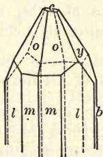
Fig. 155. Topaz
