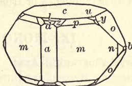
Fig. 158. Anglesite.
