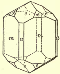
Fig. 91. Rutile.
