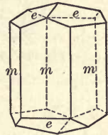
Fig. 127. Calcite.
