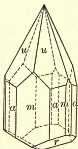
Fig. 140. Tourmaline.
