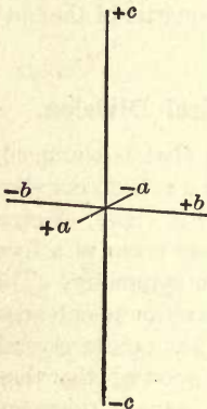
Fig. 143. Orthorhombic Axes.
