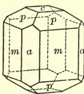
Fig. 90. Vesuvianite.
