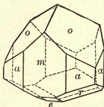
Fig. 139. Tourmaline.
