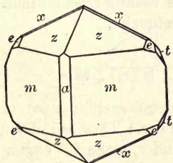
Fig. 157. Brookite.
