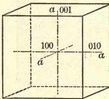
Fig. 29. Cube.
