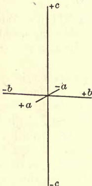
Fig. 6. Orthorhombic Crystal Axes.
