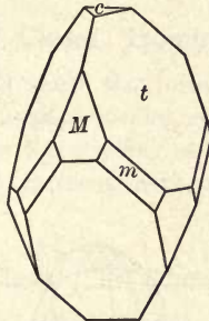
Fig. 126. Calcite.
