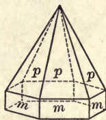
Fig. 116. Zincite.
