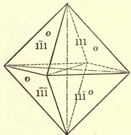
Fig. 30. Octahedron.
