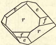
Fig. 128. Chabazite.
