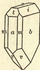
Fig. 162. Calamine.
