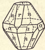
Fig. 130. Corundum.
