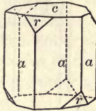
Fig. 129. Corundum.
