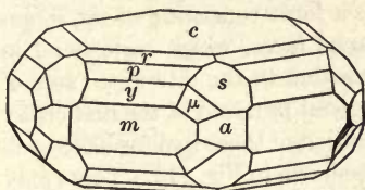
Fig. 115. Apatite.
