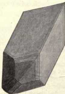
Fig. 292. Baveno Twin.
