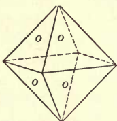
Fig. 12. Octahedron.
