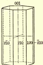
Fig. 81. Ditetragonal Prism.
