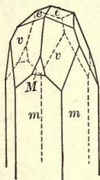
Fig. 136. Calcite.
