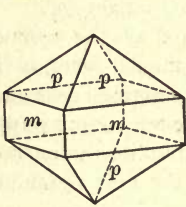
Fig. 85. Zircon.
