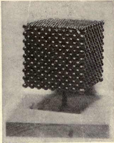
A. Cube.
