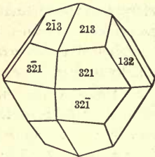
Fig. 54. Diploid.
