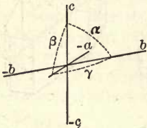
Fig. 180. Triclinic Axes.
