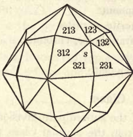
Fig. 46. Hexoctahedron.
