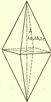
Fig. 7. Orthorhombic Pyramid.
