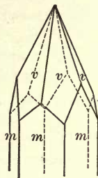
Fig. 134. Calcite.
