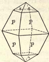
Fig. 151. Sulphur.
