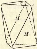
Fig. 125. Calcite.
