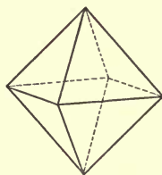
Fig. 17. Octahedron.
