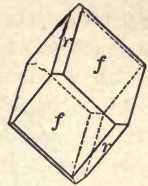
Fig. 124. Calcite.
