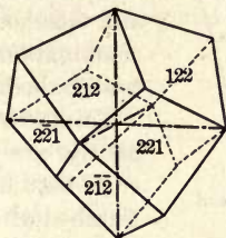
Fig. 69. Deltoïd Dodecahedron.
