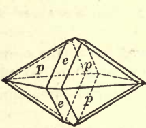
Fig. 89. Vesuvianite.
