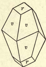
Fig. 133. Calcite.
