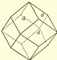
Fig. 211. Dodecahedron.
