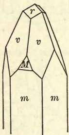
Fig. 135. Calcite.
