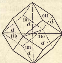
Fig. 33. Dodecahedron.
