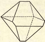
Fig. 18. Distorted Octahedron.
