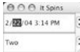
Figure 14-9. SpinnerDemo output
